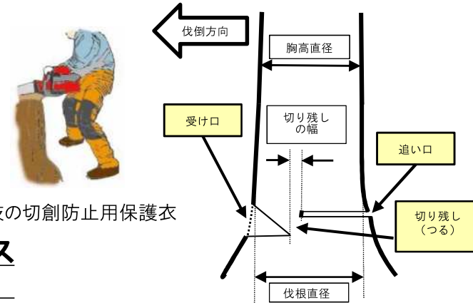
（図2）受け口、追い口等の関係図
